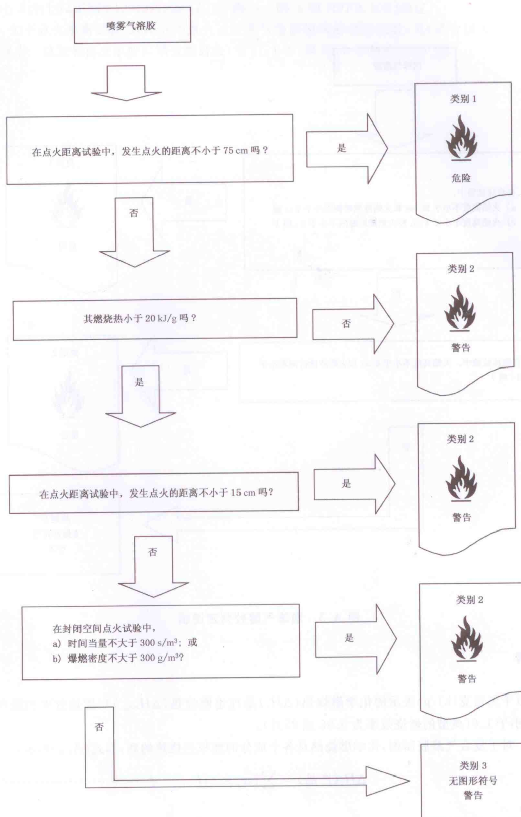
图 A.2 喷雾气溶胶判定逻辑
