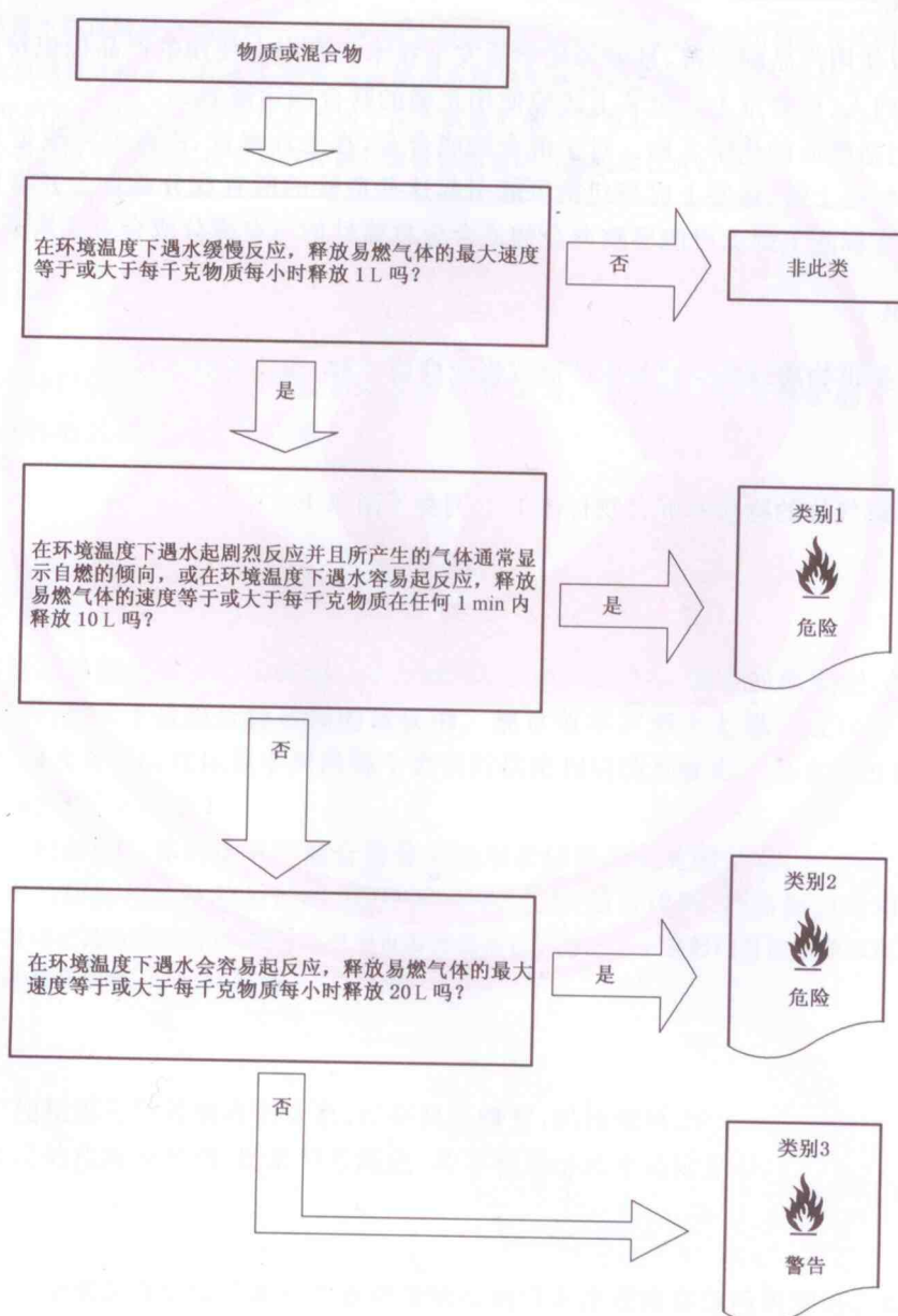
图 A.1 遇水放出易燃气体的物质和混合物判定逻辑
